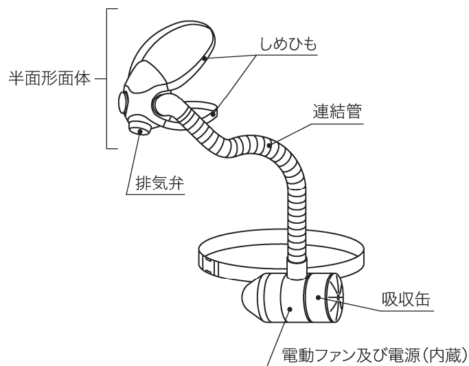
図 2－半面形面体をもつ隔離式面体形 G-PAPR の例
