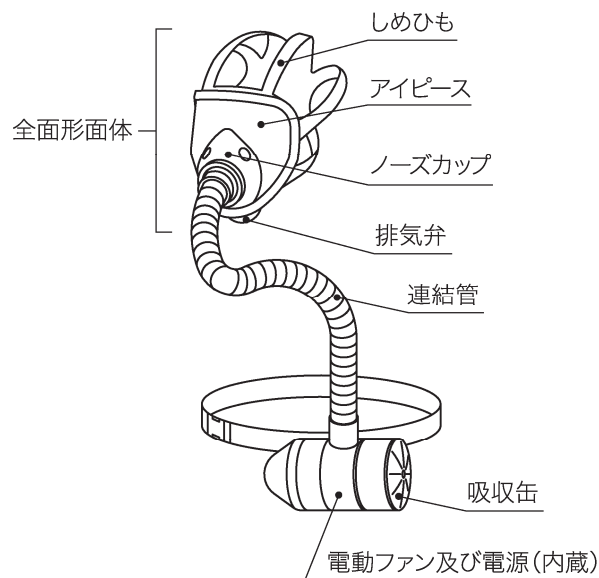
図 1－全面形面体をもつ隔離式面体形 G-PAPR の例
