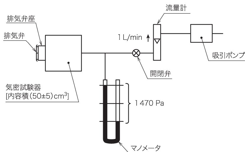
図 17—排気弁の作動気密試験装置の例
